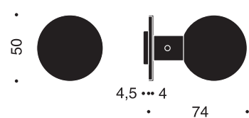
Knopdrücker Kugel
